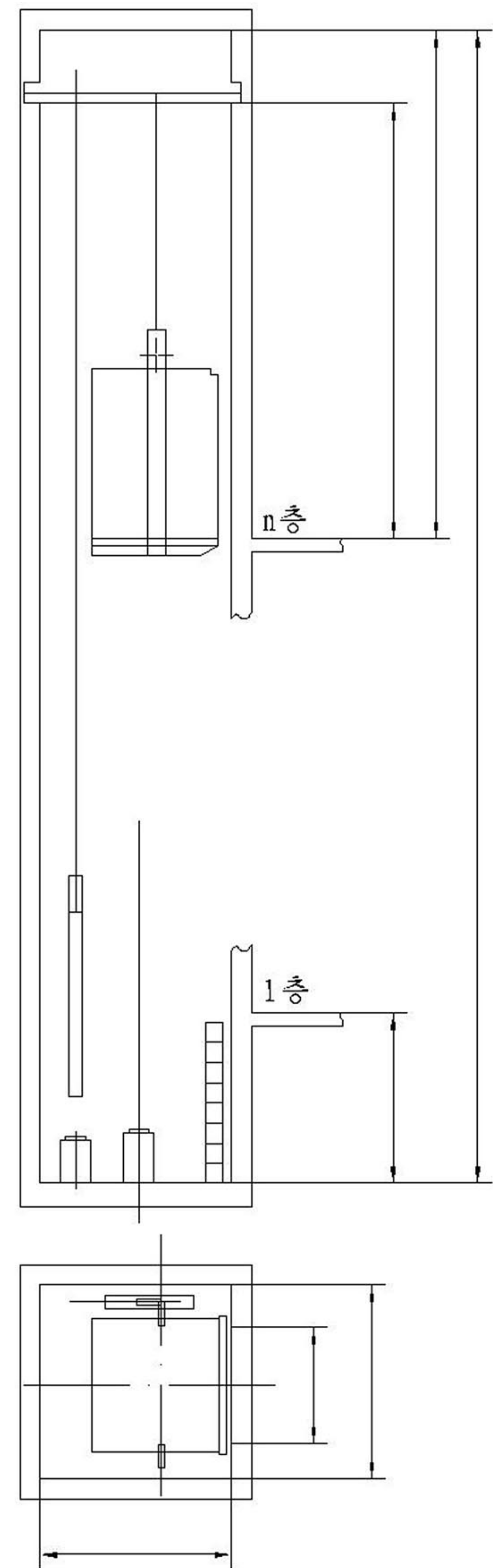
기계실이 없는 경우 WITHOUT MACHINE ROOM 无机房
